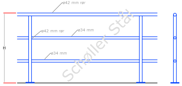
Rækværk type 1 A
